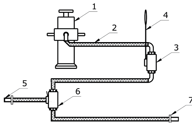
Рис. 3 Схема гидравлической системы механизма опрокидывания грузового кузова
