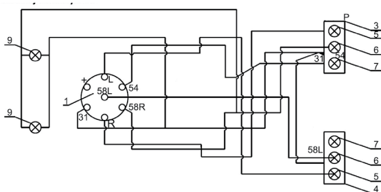
Рис. 3 Схема электрической проводки разбрасывателя 1 - вилка 7-ми-контактная, 3 - фонарь комбинированный задний правый, 4 - фонарь комбинированный задний левый, 5 - лампочки огней направления езды, 6 - лампочки задних габаритных огней, 7 - лампочки огней торможения «STOP», 8- лампочки подсветки номера, 9 - фонарь габаритный передний, 10 - габаритный фонарь.
